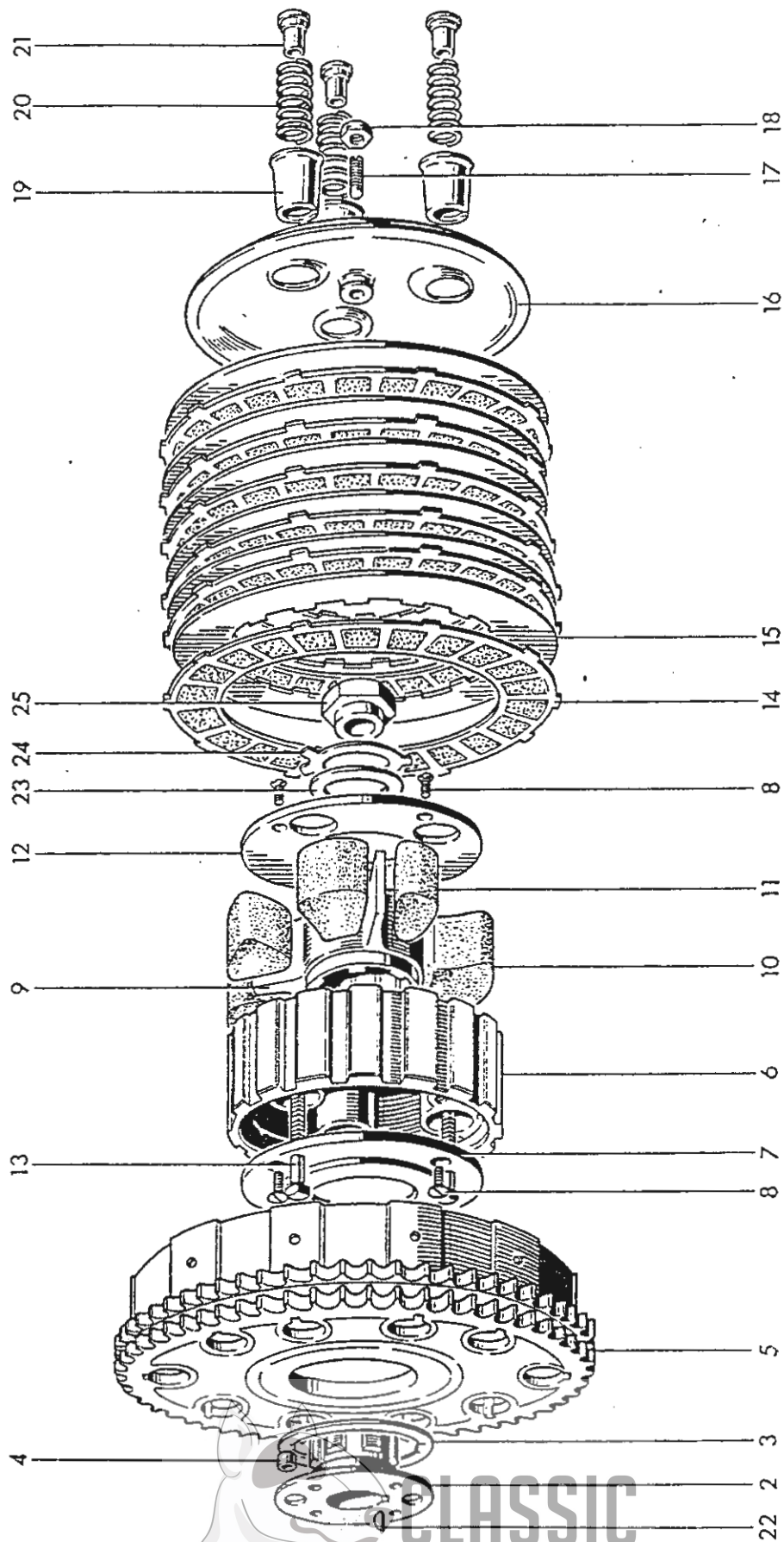
Fig. 10. CLUTCH
